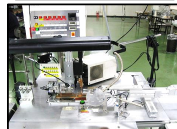
XYステージ半自動溶接機
