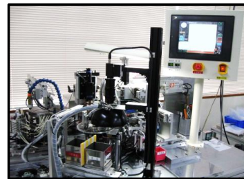
画像センサ付自動溶接機
