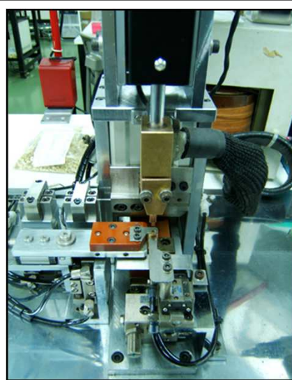
接点自動供給型半自動溶接機 2
