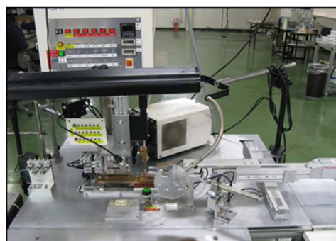
XYステージ半自動溶接機
